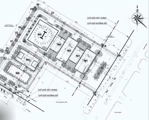
MINH HOẠ QUY HOẠCH TỔNG MẶT BẰNG TỈ LỆ: 1/500
